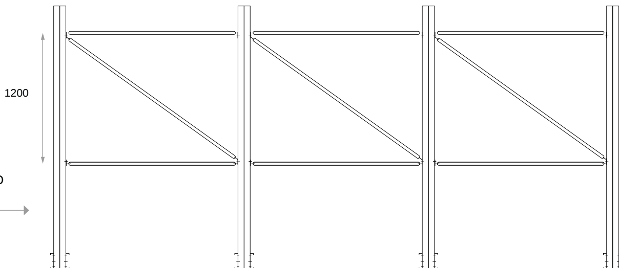
SCHEMA MONTAGGIO CROCIERE
