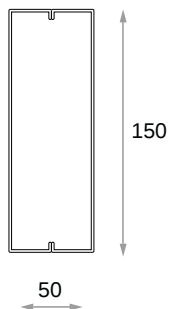
SEZIONE COLONNA
