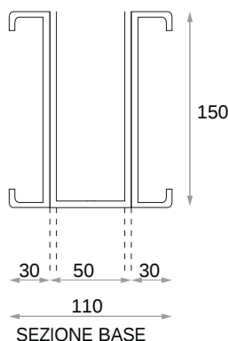
SEZIONE BASE
