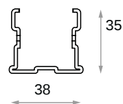
SEZIONE MONTANTE
