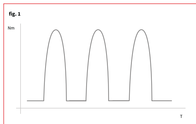
Diagramma della coppia di serraggio in un avvitatore idraulico ad impulsi.
