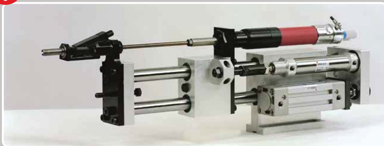
Esempio di avvitatore autoalimentato con applicazione di portainseri ed inserto filettati (per gentile concessione di MTA TECH S.r.l.) Example of self-powered screwdriver with application of bit holder and threaded insert (by kind permission of MTA TECH S.r.l.)
