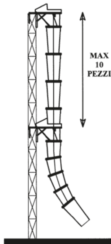
Telaio sostegno convogliatore per balcone e/o ponteggio
